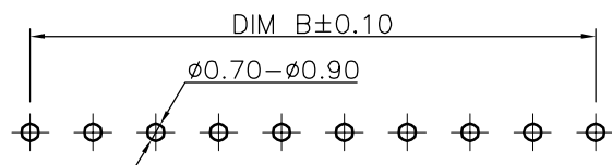
P.C.B Layout
