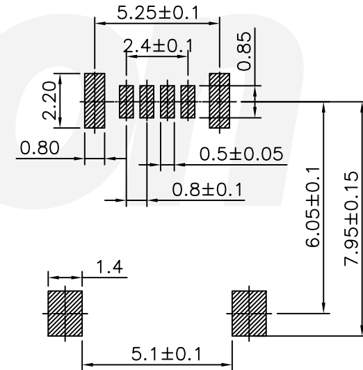
P.C.B. Layout
