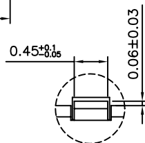
Detail:B Scale:5:1
